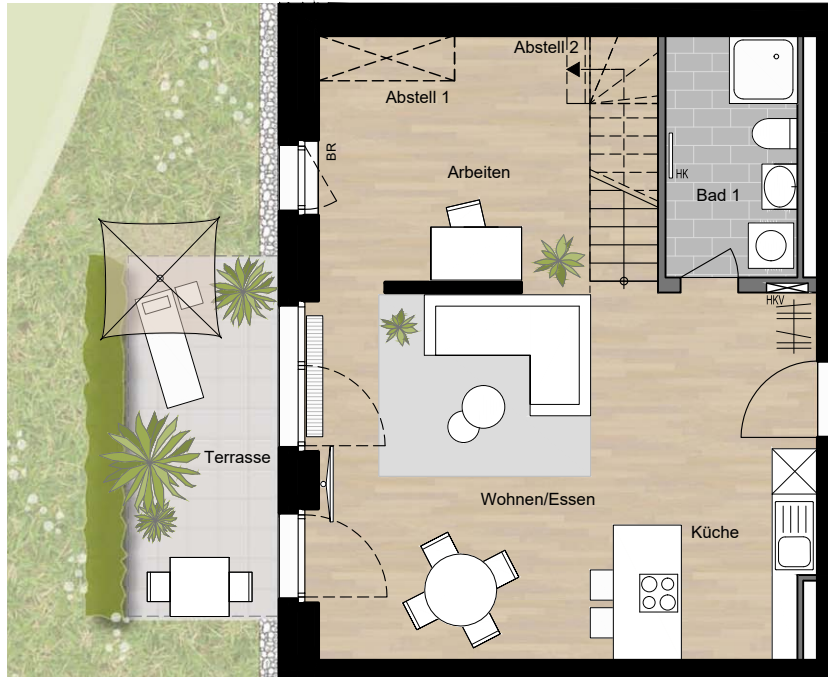
Erdgeschoss
